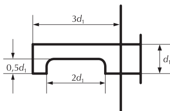
Slika 21 – Poluotvorena cijev Fig. 21 – Half-open pipe feed distributor
