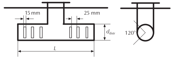
Slika 22 – T-raspodjelnik, tipične dimenzije Fig. 22 – T-feed distributor, typical dimensions
