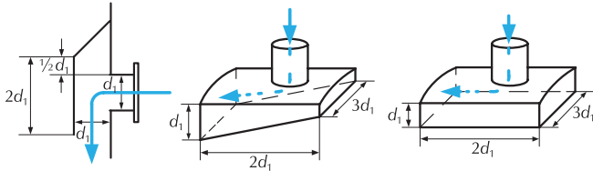
Slika 19 – Tipične dimenzije deflektora Fig. 19 – Deflector – typical dimensions
