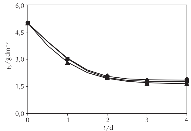
Slika 2 – Promjena koncentracije supstrata u otpadnoj vodi iz proizvodnje farmaceutika \gamma_{s0} = 5,01 \text{ g dm}^{-3} za početne koncentracije aktivnog mulja X1 (◆), X2 (■), i X3 (▲) u pokusu P2 tijekom četiri dana. Usporedba rezultata pokusa i modela (—)
