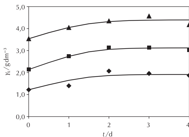
Slika 5 – Promjene koncentracija aktivnog mulja X1 (◆), X2 (■), i X3 (▲) u pokusu P2 tijekom četiri dana. Usporedba rezultata pokusa i modela (—)
