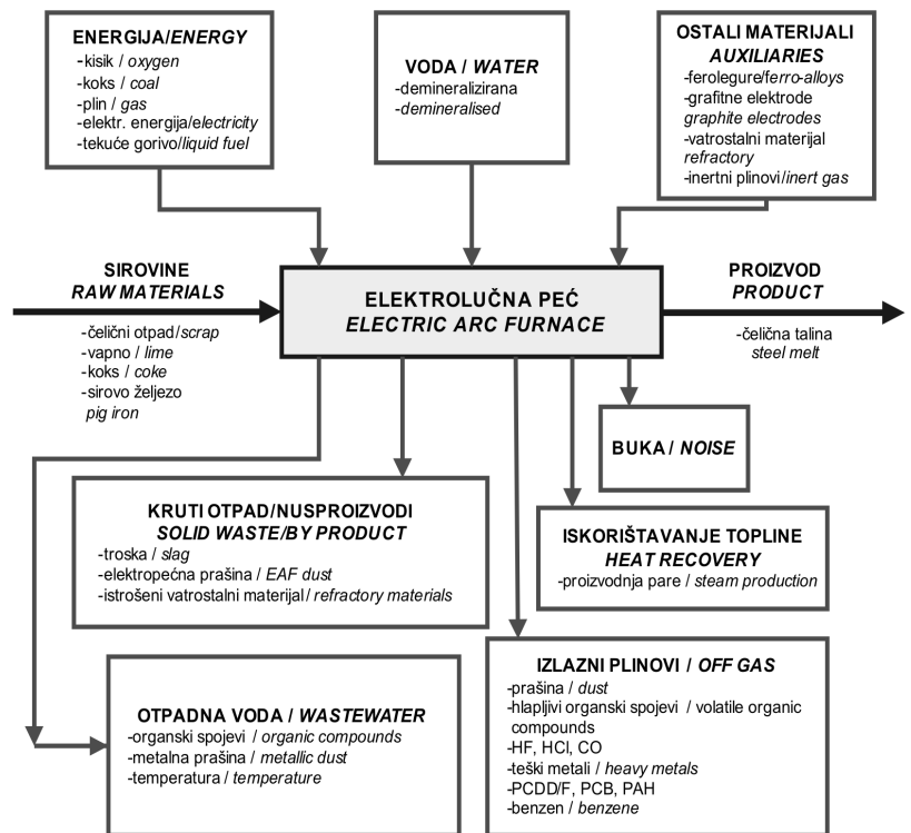
Slika 1 – Elektrolučna peč – tijek tvari i energije
